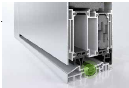
Aluminium-Verbund-Schwelle
